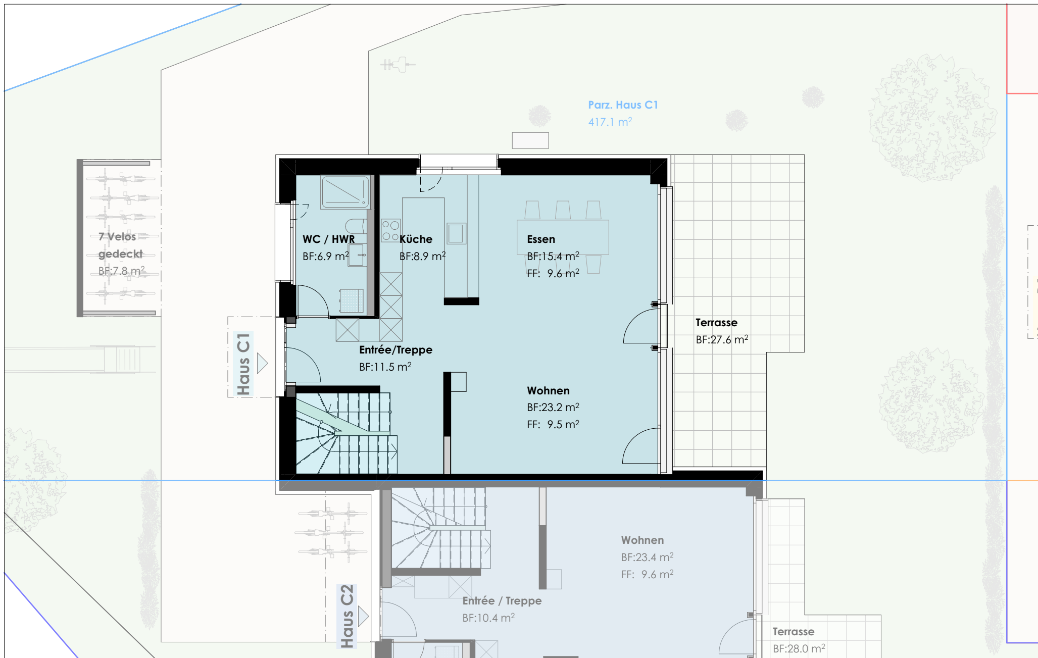
Haus C1 Grundriss Erdgeschoss
