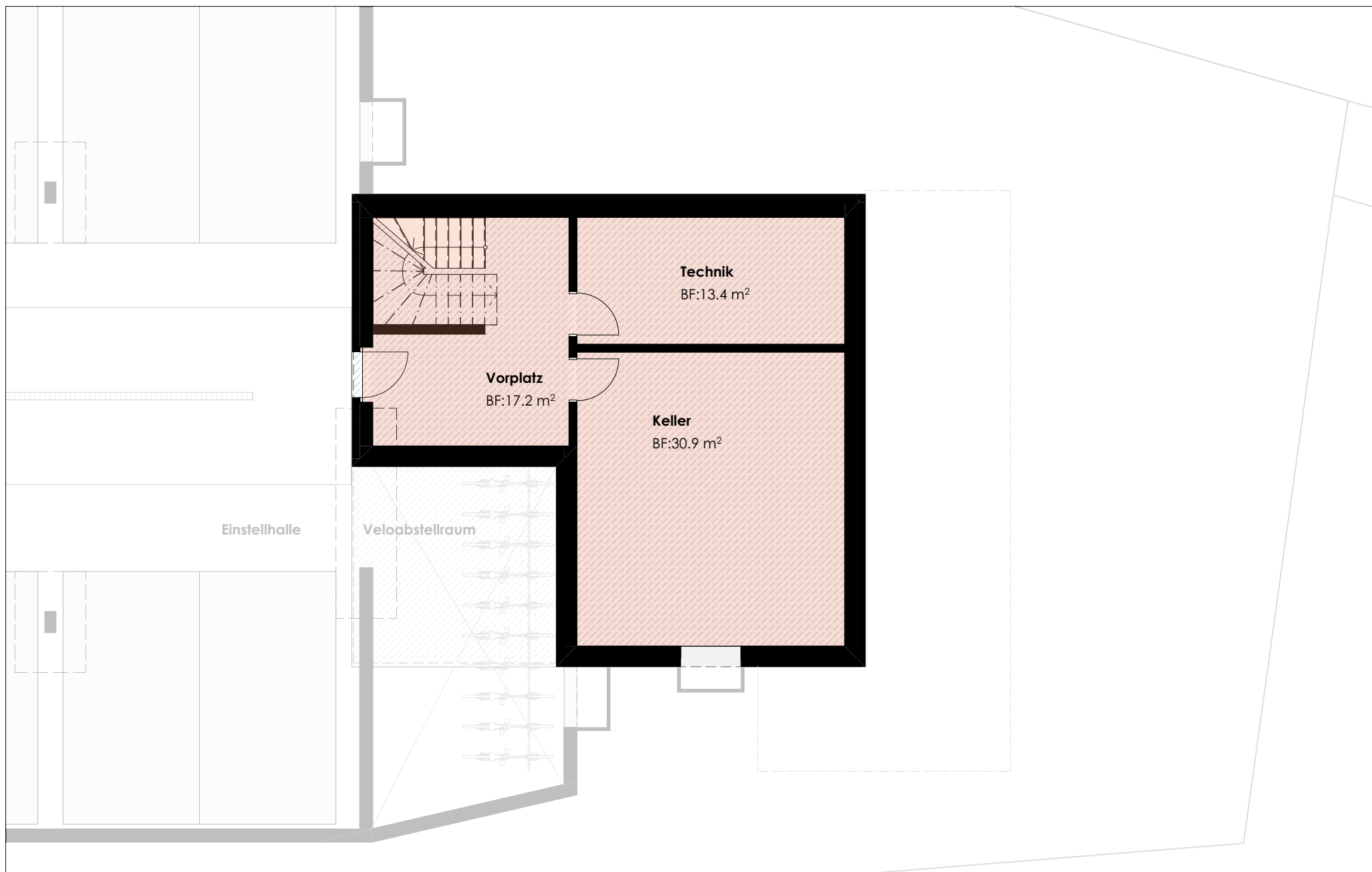
Haus A Grundriss Untergeschoss
