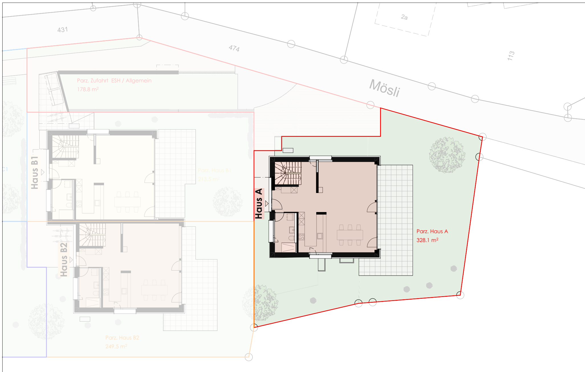
Haus A Grundriss EG mit Umgebung
