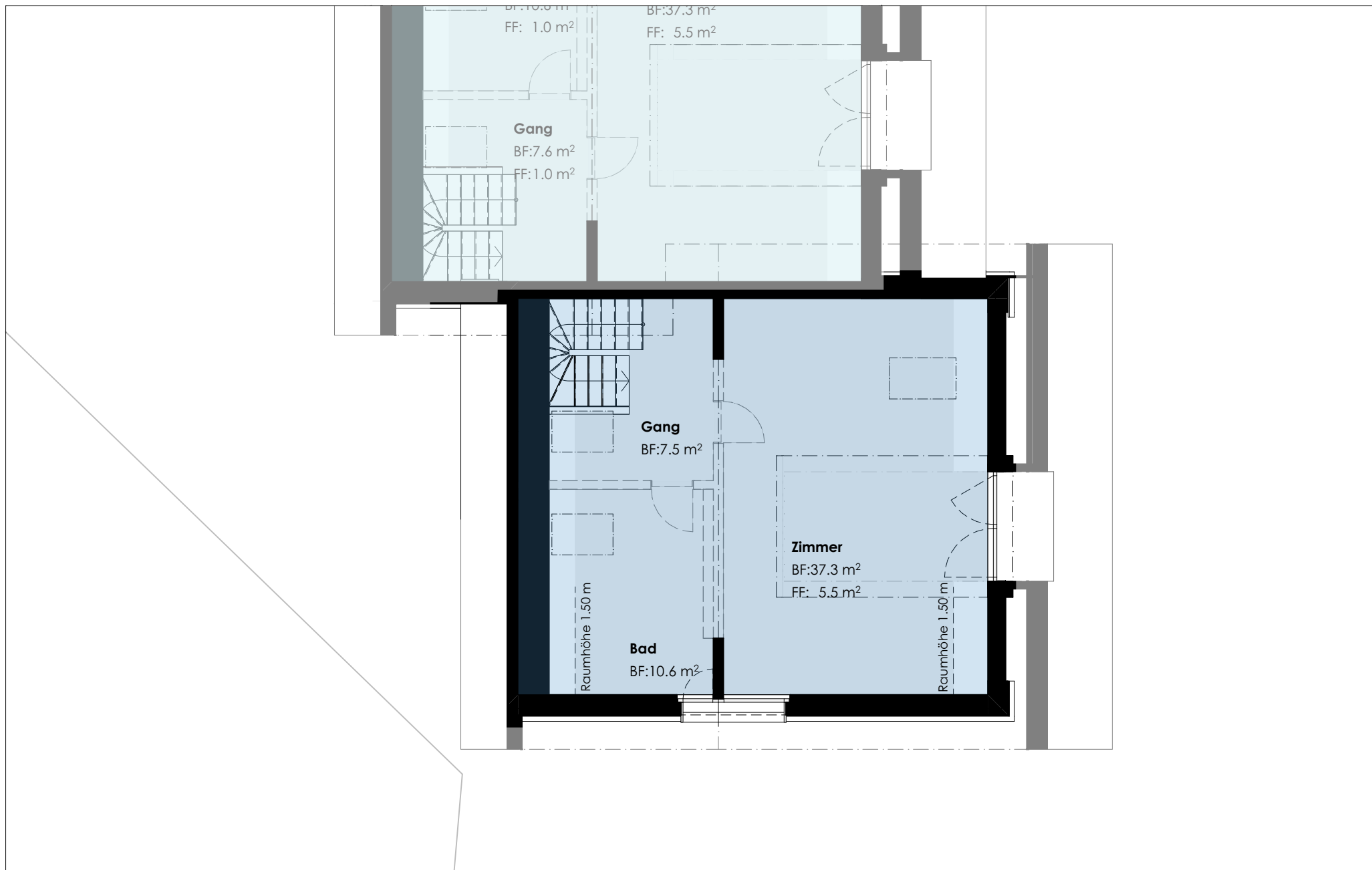
Haus C2 Grundriss Dachgeschoss (nicht ausgebaut)
