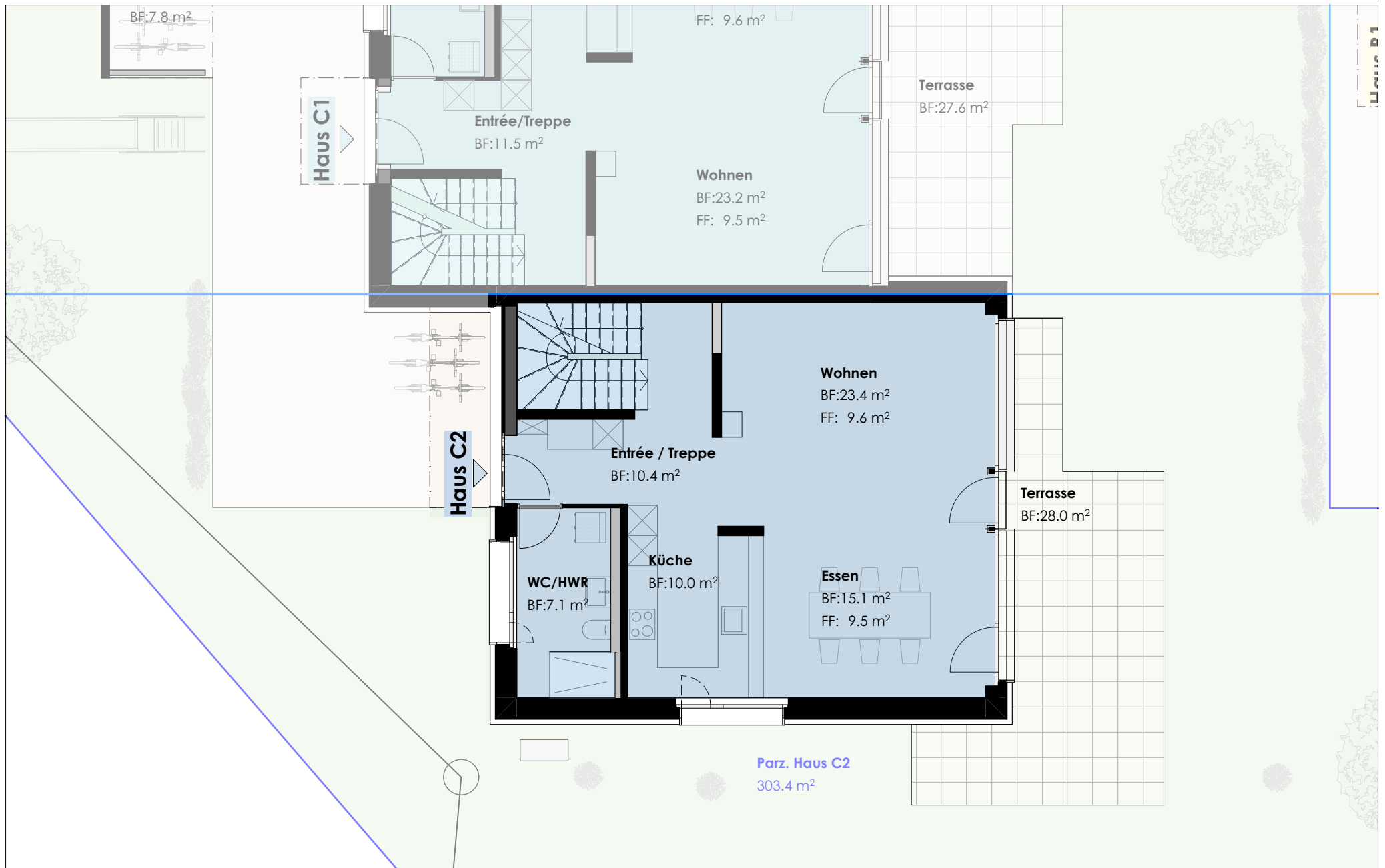
Haus C2 Grundriss Erdgeschoss
