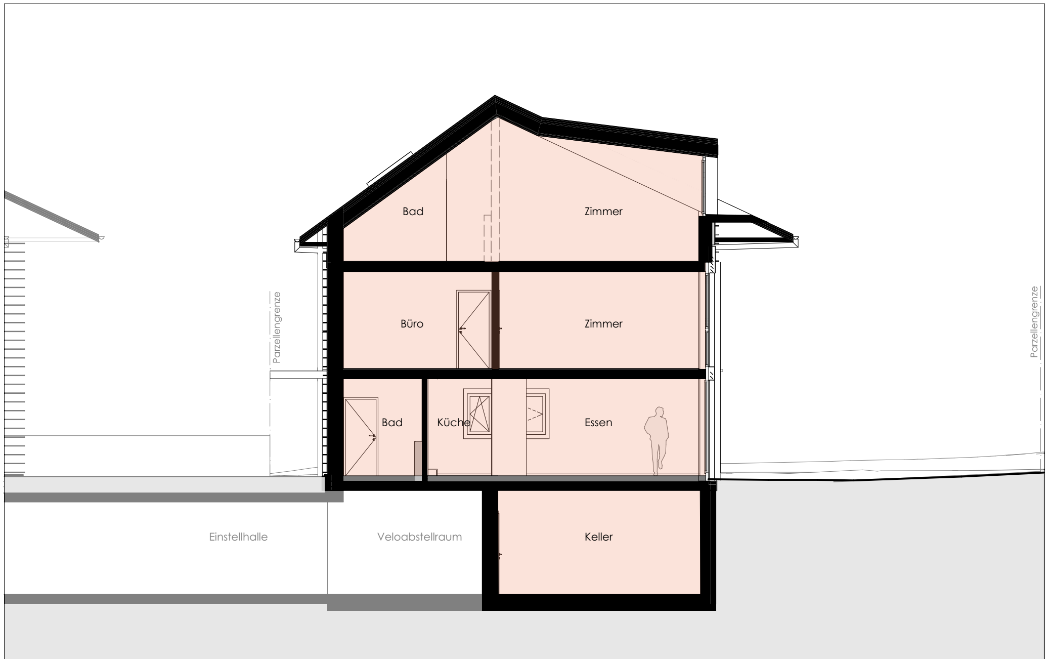
Haus A Querschnitt
