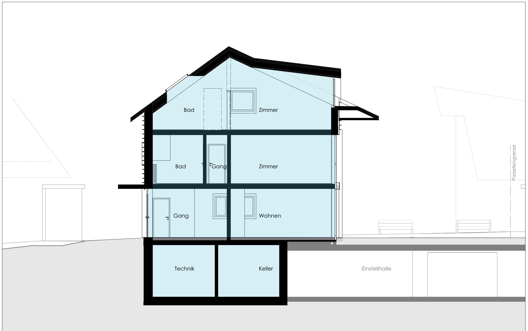
Haus C1 Querschnitt
