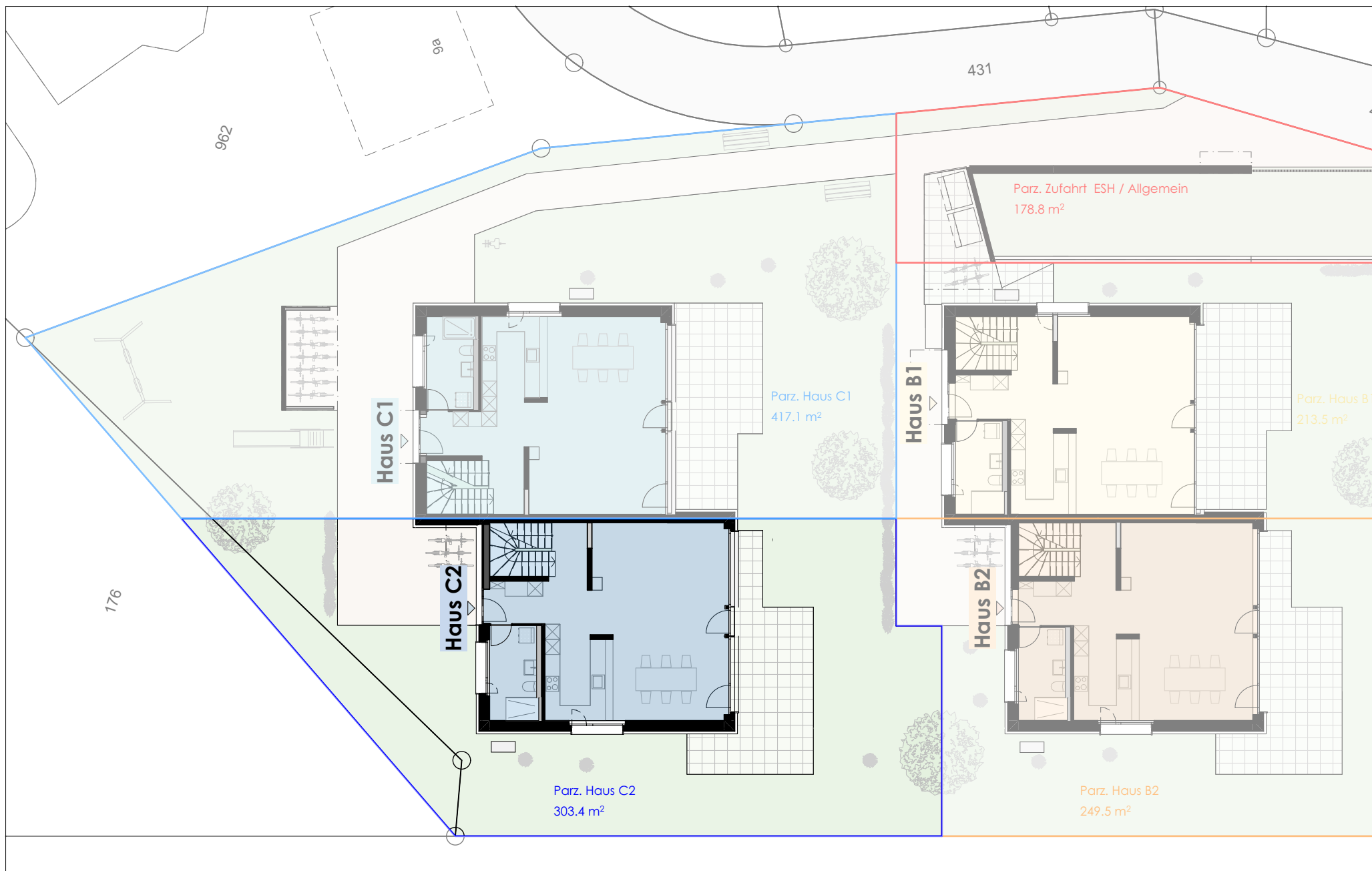
Haus C2 Grundriss EG mit Umgebung
