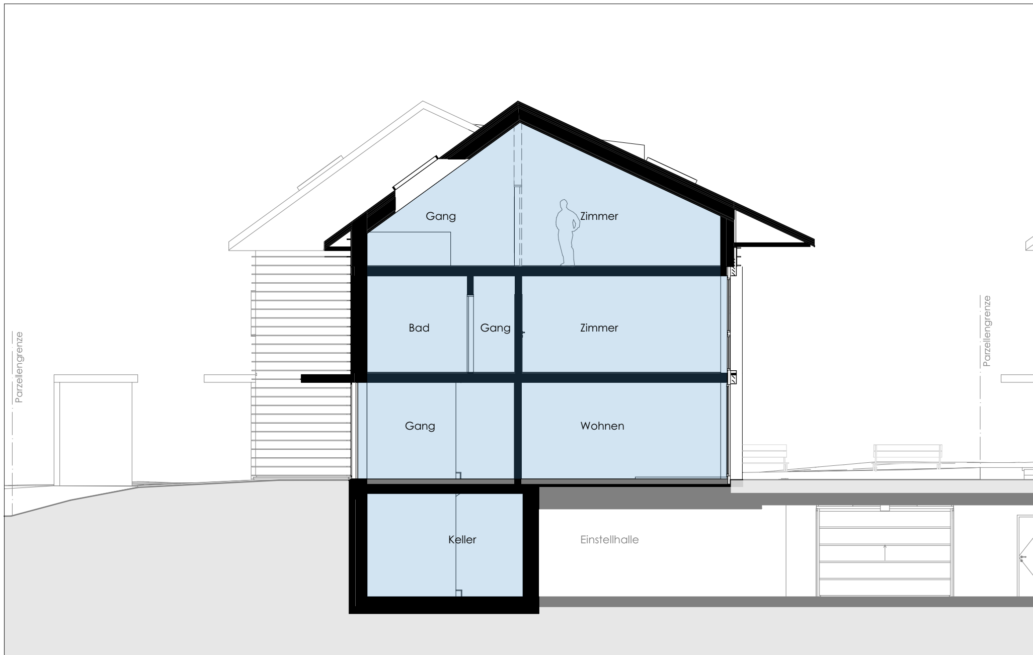
Haus C2 Querschnitt
